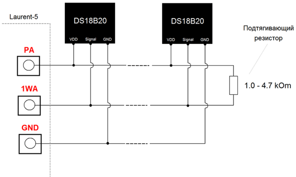
Рис. Типовая Схема подключения датчиков DS18B20 к каналу 'А' шины I-Wire модуля Laurent-5 / 5G. Величина сопротивления подтягивающего резистора зависит от длины шины (чем больше длина трассы – тем меньше сопротивление), ее топологии, кол-ва датчиков на шине и т.д. Вариант подключения к каналу 'В' шины I-Wire модуля аналогичен (используются клеммы PB, 1WB, GND).
