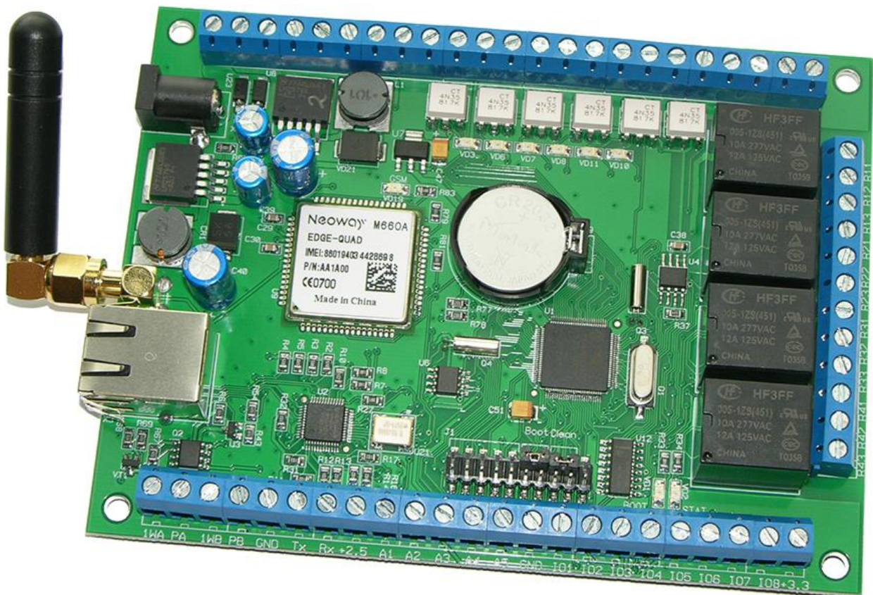
Рис. Laurent-5G с подключенной антенной KG-25.
