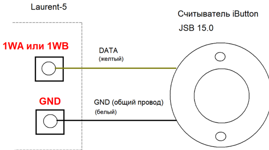
Рис. Схема подключения считывателя iButton JSB 15.0 к модулю. Линию данных следует подключить либо к клемме 1WA (если используем канал 'A' I-Wire модуля) либо к 1WB (канал 'B').
