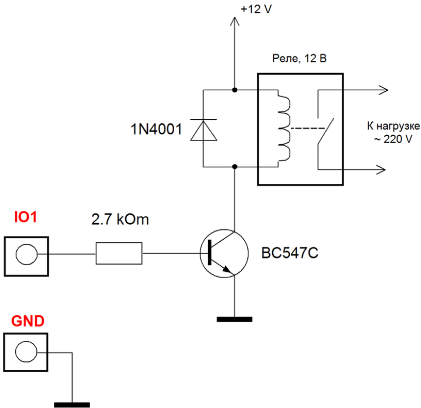
Рис. Подключение внешнего электромагнитного реле на 12 В через транзистор к линии IO настроенной “на выход”.
