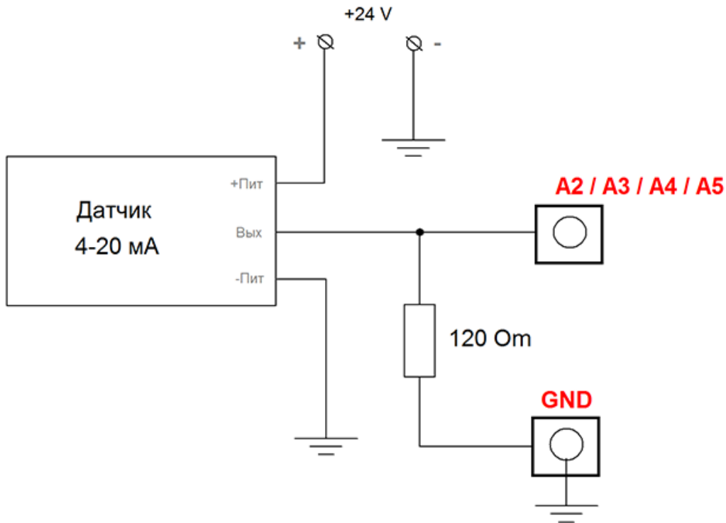
Рис. Общая схема подключения датчиков “токовая петля” к каналам АЦП А2-А5
