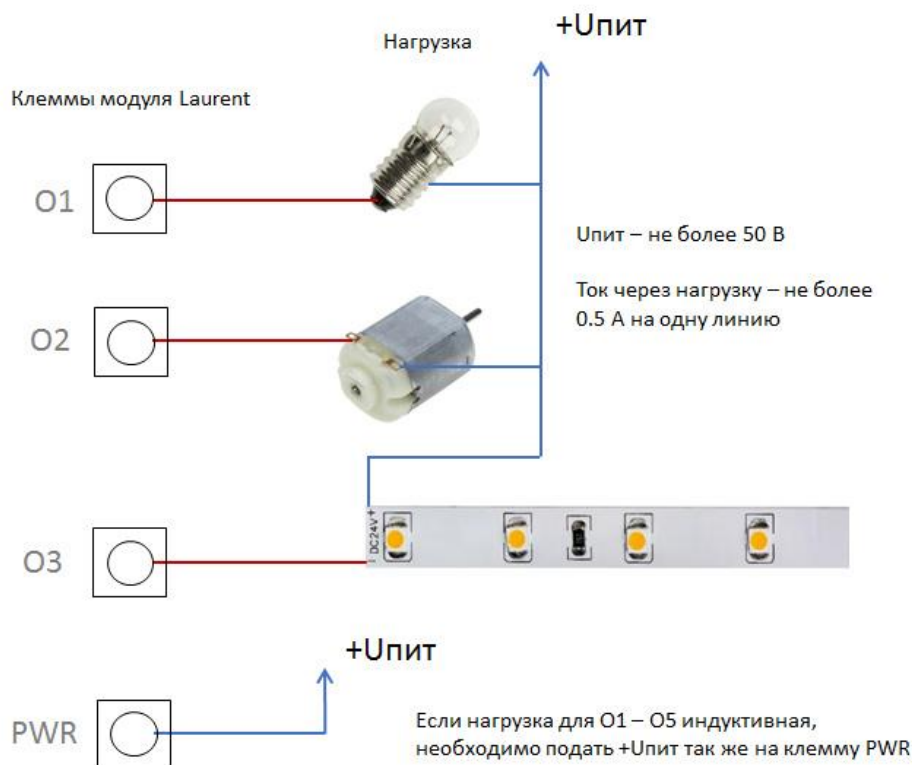
Рис. Схема подключения нагрузки для ШИМ управления к выходным силовым линиям O1 – O4.
