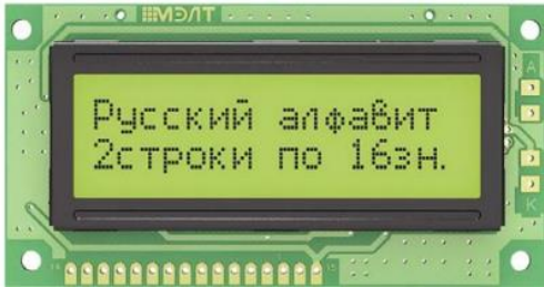
Рис. LCD дисплей MT-16S2H-2YLG компании МЭЛТ
