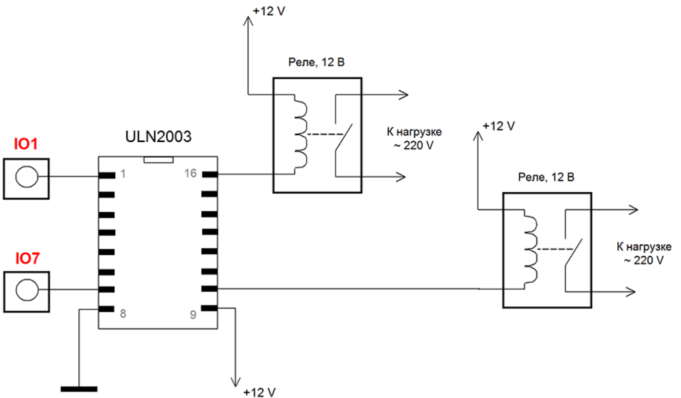
Рис. Подключение внешних электромагнитных реле на 12 В через микросхему ULN2003 (сборка транзисторов Дарлингтона) к линиям IO настроенным “на выход”.
