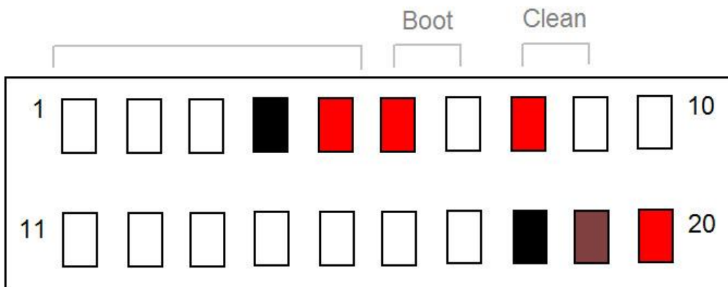
Рис. Наименование контактов “штырькового” разъема модуля Laurent-5 / 5G (вид сверху)
