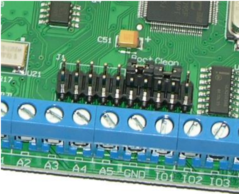
Рис. Фотография разъема J1 на плате модуля Laurent-5G
