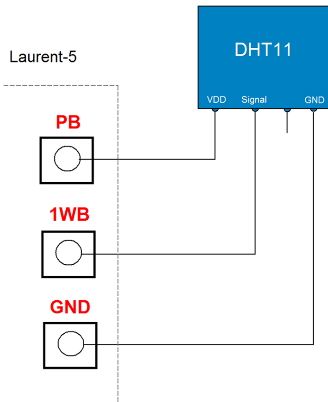
Рис. Типовая Схема подключения датчика DHT-11 / DHT-22 к каналу ‘B’ шины I-Wire модуля Laurent-5 / 5G.
