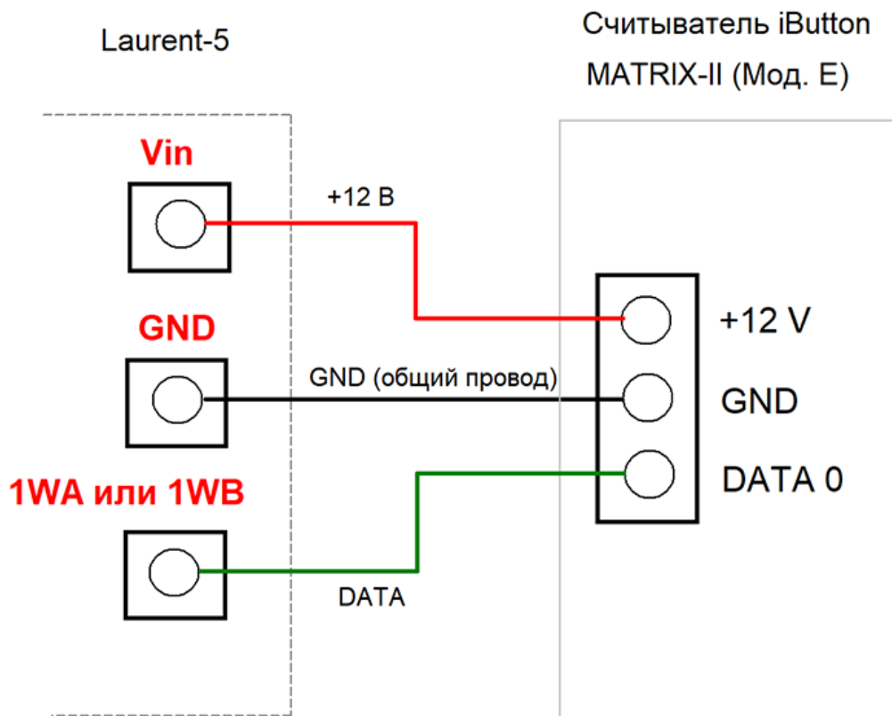
Рис. Схема подключения RFID считывателя с эмуляцией iButton MATRIX-2 (модель E). Линию данных следует подключить либо к клемме 1WA (если используем канал 'A' I-Wire модуля) либо к 1WB (канал 'B'). Питание считывателя MATRIX поступает от клеммы модуля Laurent-5/5G VIN на которую подано напряжение питания +12 В.
