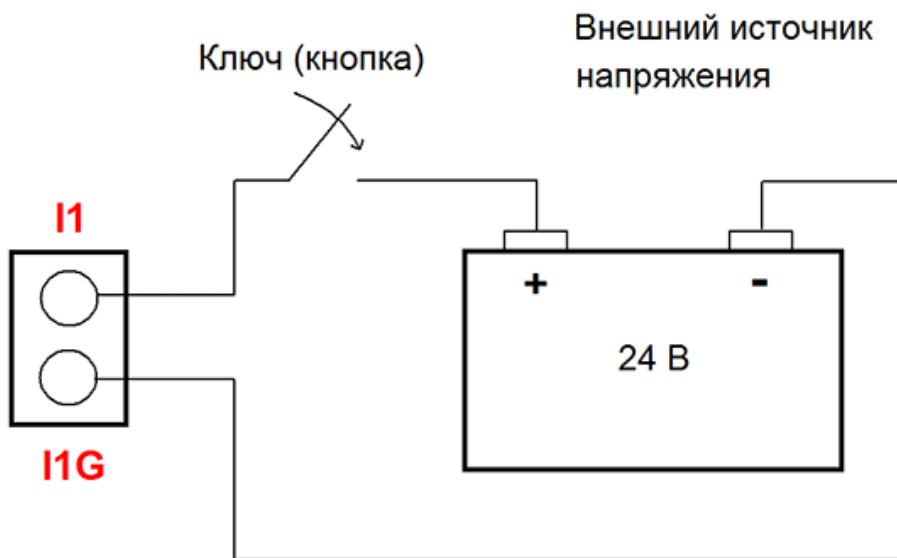
Рис. Источник сигнала (в данном случае – обычный аккумулятор, например установленный на грузовом автомобиле) для входной линии IN_1 “развязан” относительно самой платы (ее источника питания).
