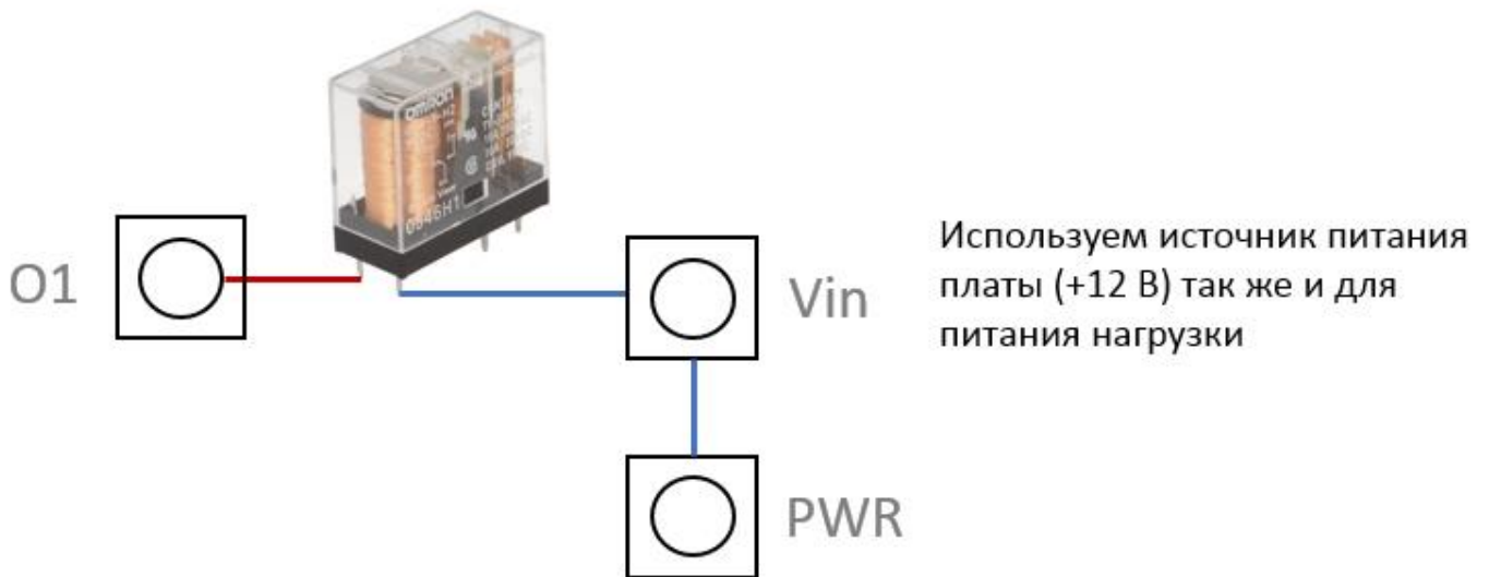
Рис. Подключение внешнего реле на +12 В. Предположим, что питание самого модуля осуществляется источником на 12 В. Тогда внешнее реле так же будем питать от этого же источника (входное напряжение +12 В возьмем с клеммы Vin).
