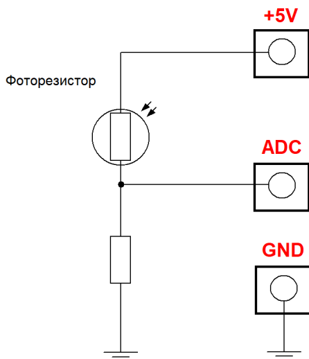
Рис. Схема измерения степени освещенности с использованием фоторезистора включенного в плечо делителя напряжения.
