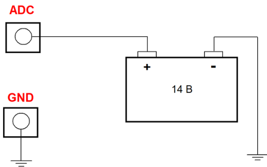
Рис. Простая схема измерения напряжения аккумуляторной батареи.
