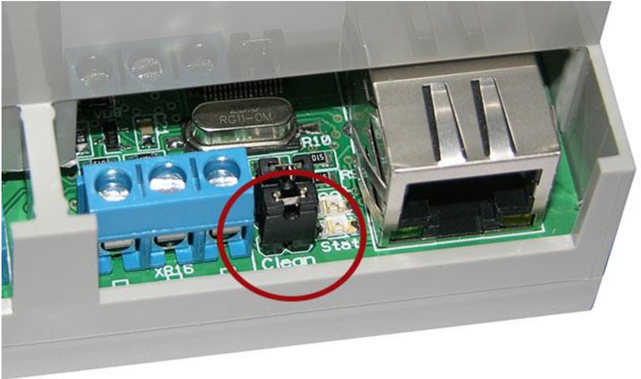
Рис. Джампер сброса настроек Clean модуля Laurent-2D .
