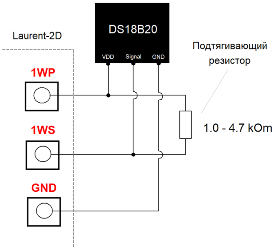
Рис. Типовая Схема подключения датчика DS18B20 к шине 1-Wire модуля Laurent-2D. Подтягивающий резистор может потребоваться при относительно больших длинах кабеля от модуля до датчика (10-20 метров и более). Величина сопротивления подтягивающего резистора зависит от длины шины (чем больше длина трассы – тем меньше сопротивление).
