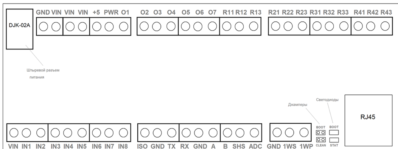
Рис. Расположение и наименование клеммных разъемов модуля Laurent-2D
