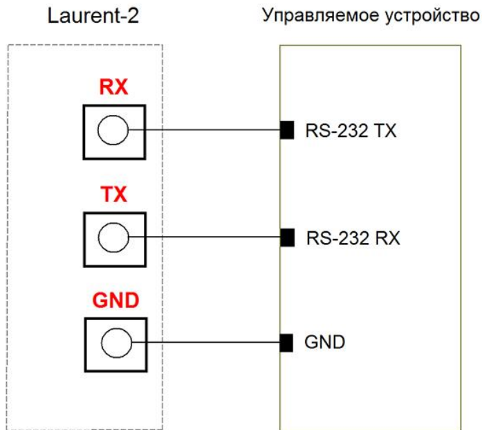
Рис. Схема подключения устройств с интерфейсом RS-232 к модулю Laurent-2D
