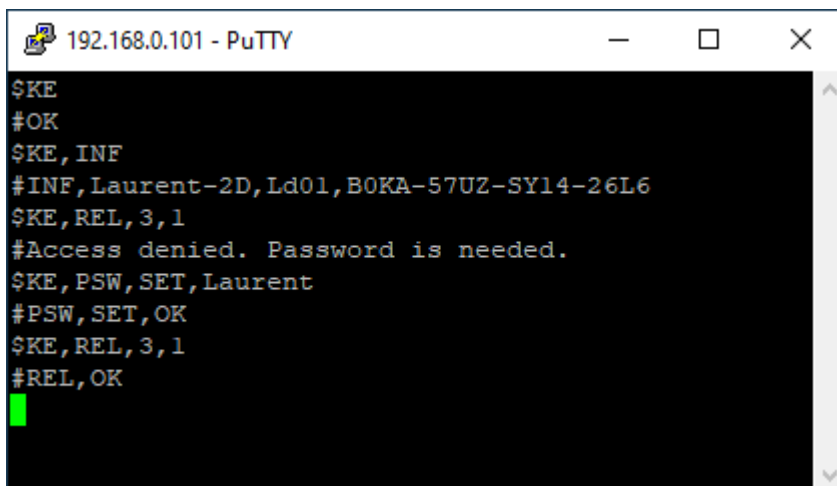
Рис. Обмен Ке-командами через терминал putty
