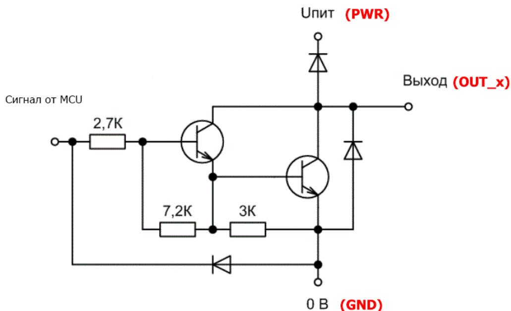
Рис. Схема электрическая выходного каскада силовой линии OUT модуля Laurent-2D (микросхема ULN2003 ). Подключение клеммы модуля PWR (общий вывод для всех линий OUT1-OUT7 ) к плюсу источника питания нагрузки (защитный диод к коллектору транзистора) позволит минимизировать негативные эффекты от ЭДС самоиндукции, возникающей в момент отключения индуктивной нагрузки (реле или электродвигателя).
