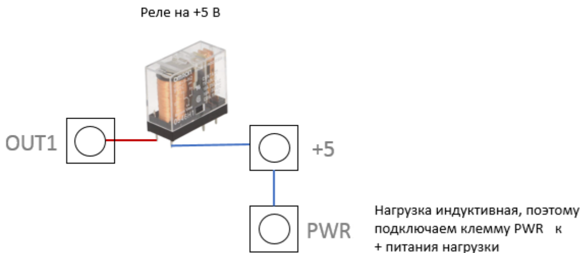
Рис. Подключение внешнего реле на +5 В. Питание для нагрузки (реле) берем с самой платы Laurent-2D (клемма +5 – пятивольтовый источник напряжения от внутреннего стабилизатора).
