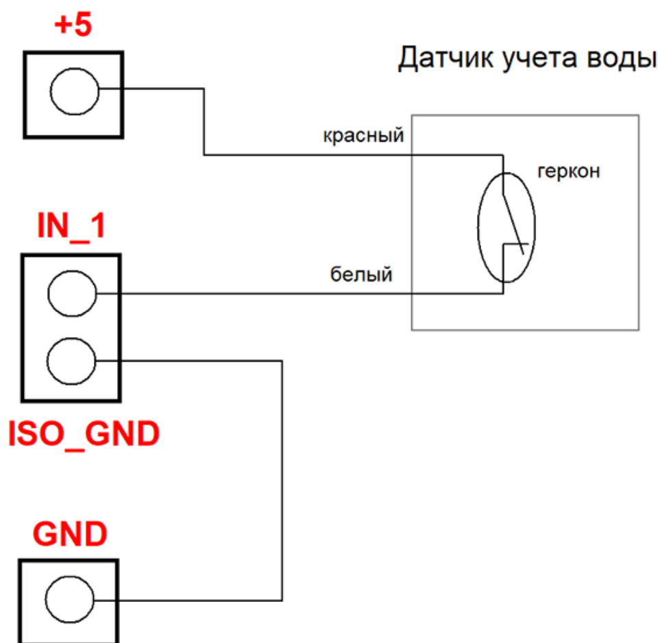
Рис. Схема подключения счетчика воды с импульсным выходом к входной оптоизолированной линии IN_1 для подсчета входящих импульсов, которые можно будет пересчитать в расход воды в м 3
