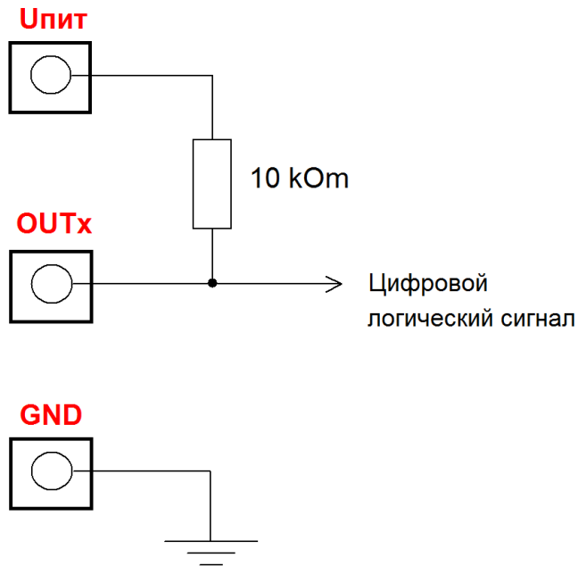
Рис. В том случае, если необходимо формировать цифровой логический сигнал с помощью линий OUT – достаточно линию OUT “подтянуть” через резистор к плюсу источника питания (+5, V_{in} ). Сигнал будет инвертированный.
